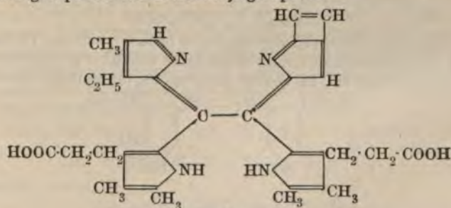
Hæmoporphyrin, \text{C}_{33}\text{H}_{36}\text{O}_4\text{N}_4 .
